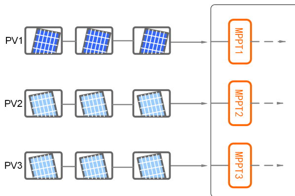
Figura 5-3 Configuração de entrada FV
