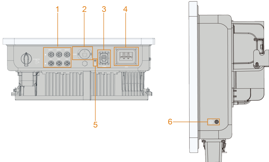
Figura 5-1 Terminais (SG10RS-L2, por exemplo)
