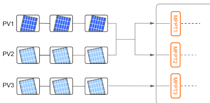
Figura 5-5 Conexão paralela parcial Apenas
