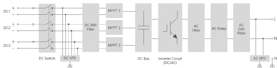
Figura 2-4 Diagrama do circuito (SG10RS-L2, por exemplo)
