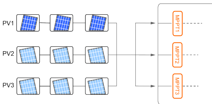
Figura 5-4 Conexão paralela
