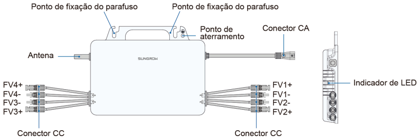
Figura 3-2 Design externo
