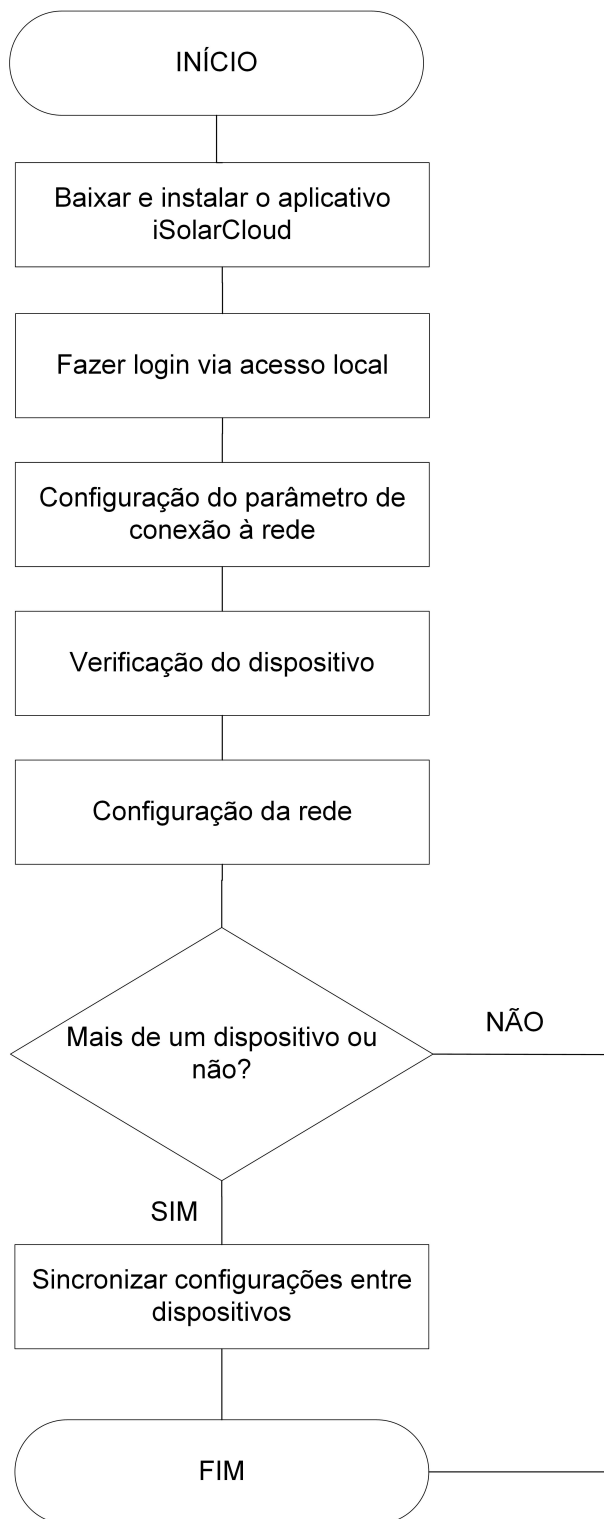
Figura 5-2 Gráfico do fluxo de configuração da operação de conexão à rede
