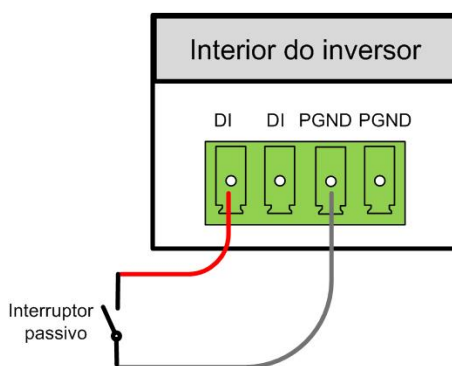
Figura 5-9 Contato de parada local
