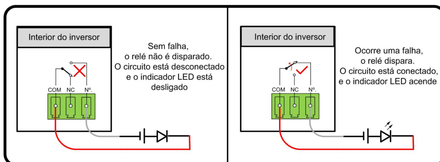
Figura 5-7 Contato normalmente aberto
