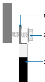
Figura 5-3 Conexão do cabo de alumínio
