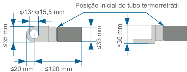
Figura 5-4 Especificações do terminal OT/DT crimpado
