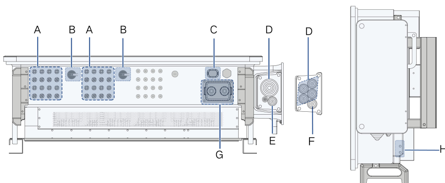
Figura 5-1 Descrição do terminal (SG50CX-P2-LV)
