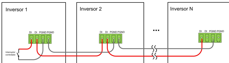
Figura 5-10 Topologia da forma encadeada
