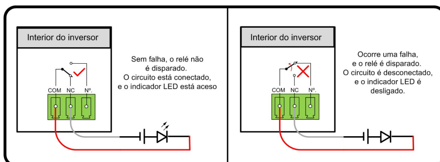
Figura 5-8 Contato normalmente fechado
