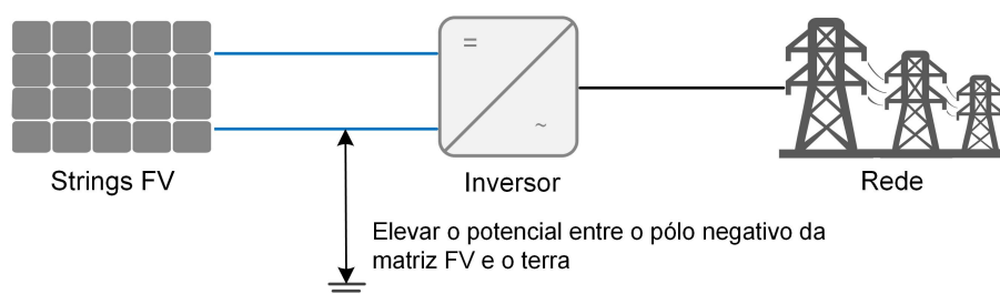
Figura 2-6 Esquema de recuperação de PID
