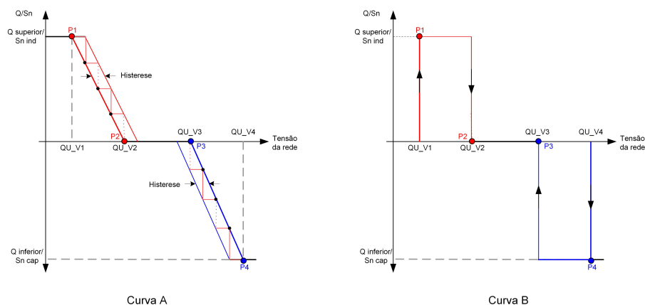
Figura 7-19 Curva de regulação de potência reativa no modo Q(U)
