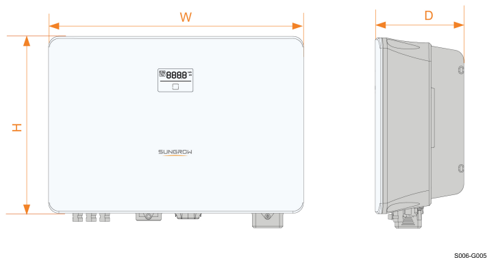
Figura 2-3 Dimensões do inversor
