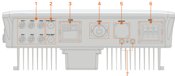
Figura 5-1 Terminais
