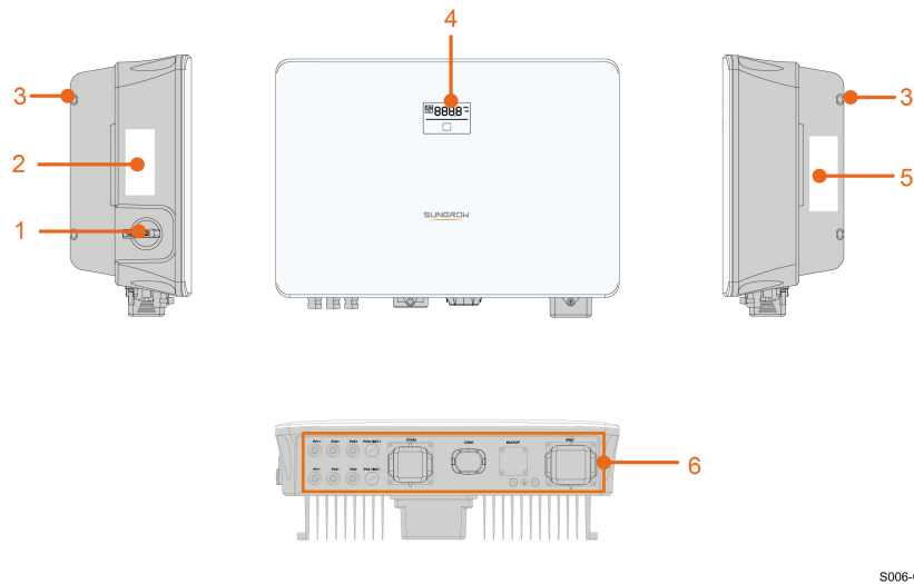
Figura 2-2 Aparência do inversor
