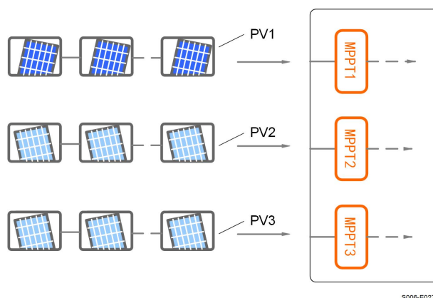
Figura 5-3 Configuração de entrada FV
