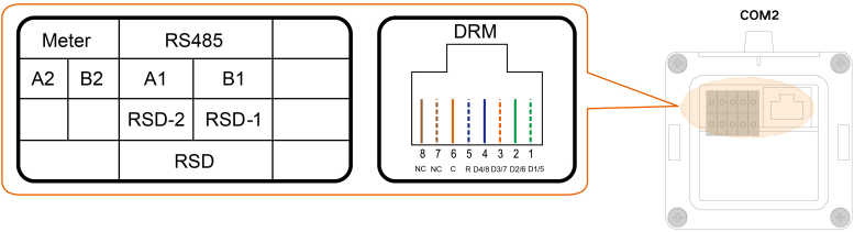
Figura 5-2 Etiqueta do terminal COM2
