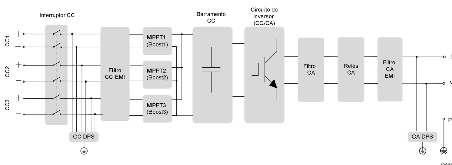
Figura 2-5 Diagrama do circuito (SG10RS por exemplo)
