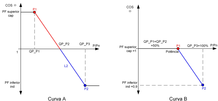
Figura 7-18 Curva de regulação de potência reativa no modo Q(P)
