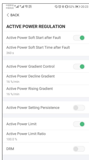
Figura 7-16 Regulação de potência ativa
